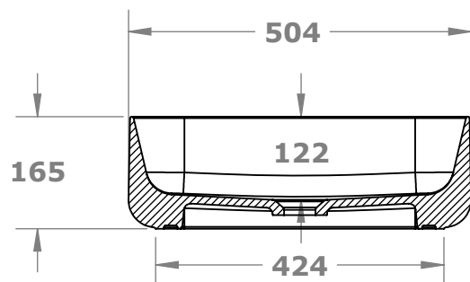
SEZIONE B-B
